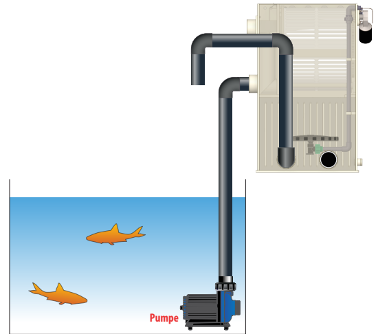
Beispiel pumpengespeiste Installation
