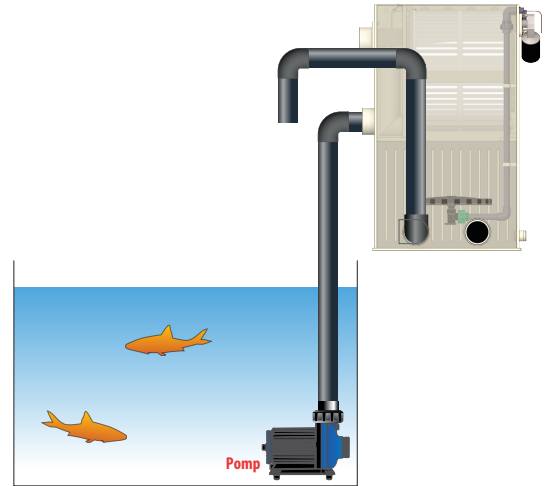
Voorbeeld pompagevoede opstelling
